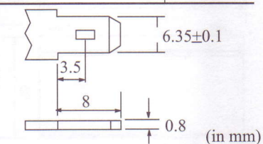
Optional Terminal F2(Fasten Tab No.250A)
